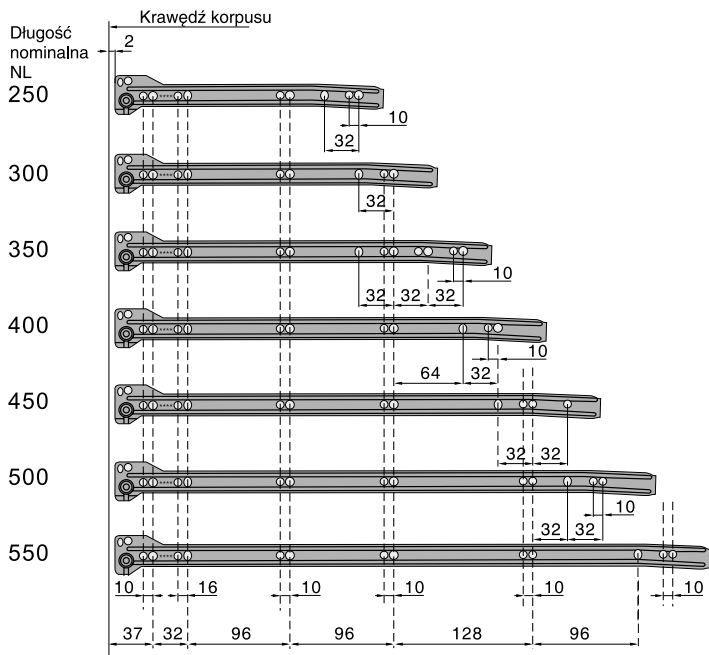
Wymiary dna
