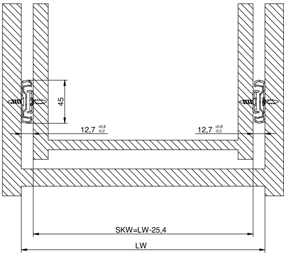
Pozycje mocowania prowadnic do korpusu
