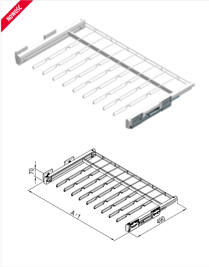
Szuflada na spodnie L-480
