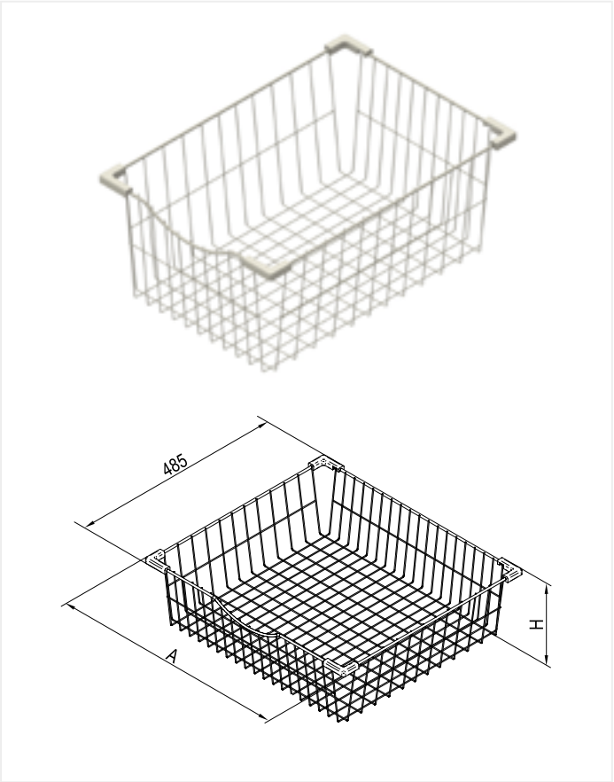
Szuflada Simpla L-500
