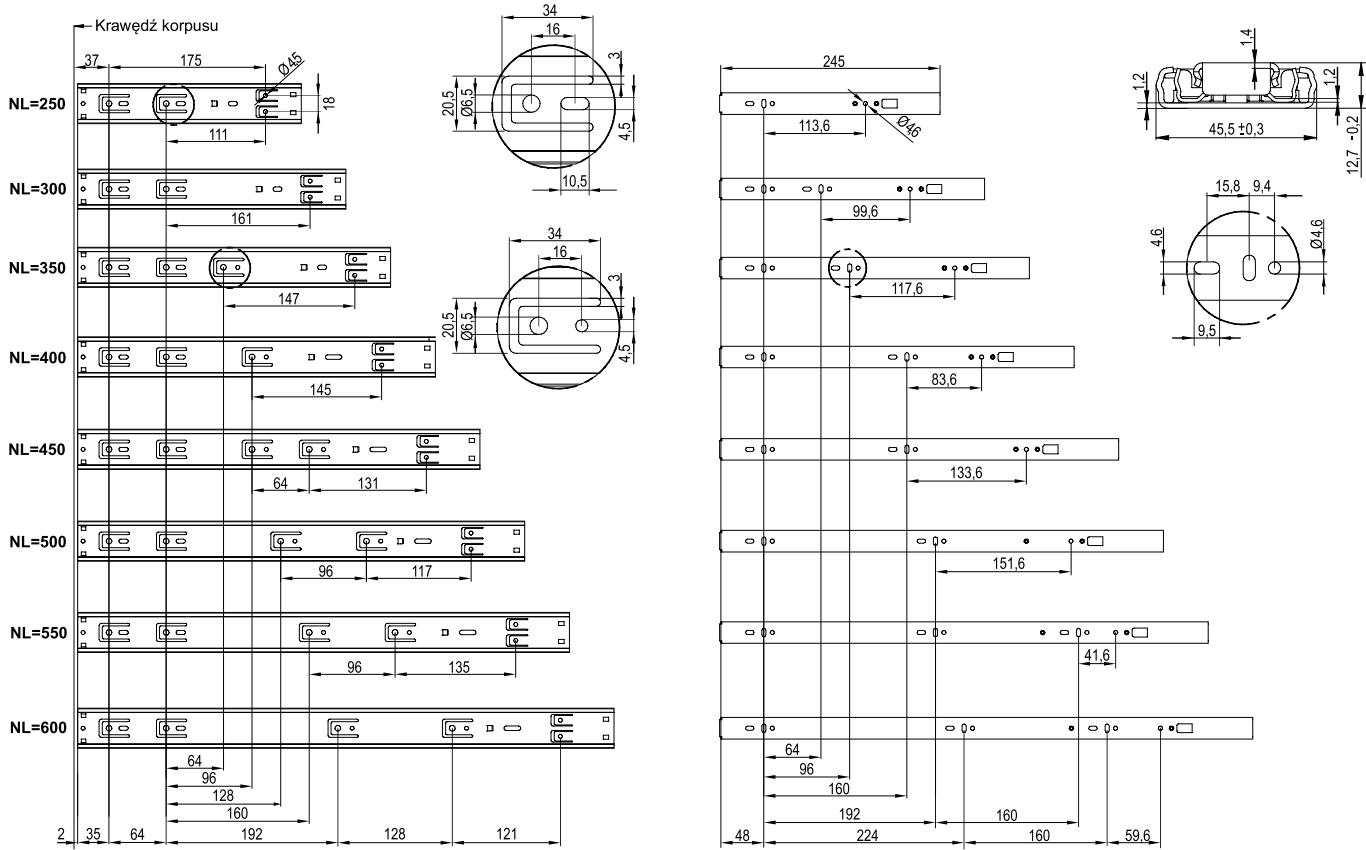
Pozycje mocowania prowadnic do korpusu
