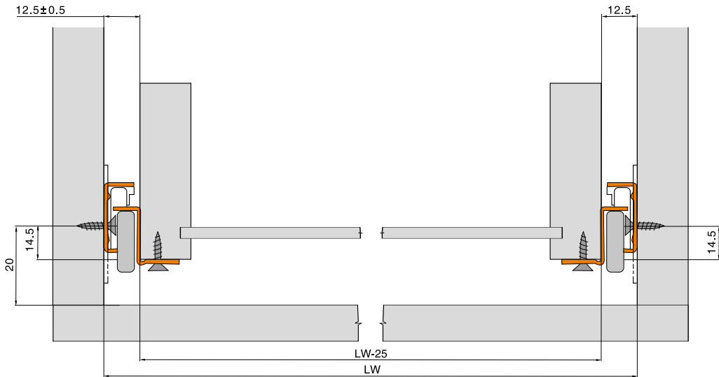
Pozycje mocowania prowadnic do korpusu
