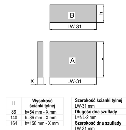
Wymiary dna i ścianki tylnej dla płyty 16 mm
