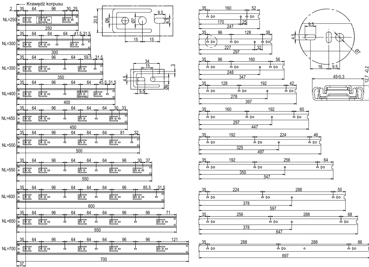
Pozycje mocowania prowadnic do korpusu
