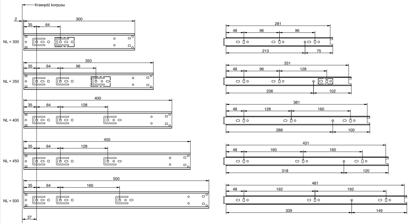
Pozycje mocowania prowadnic do korpusu
